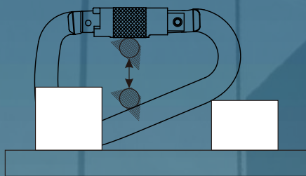
RESISTENCIA EN EJE MENOR: 7 kN
