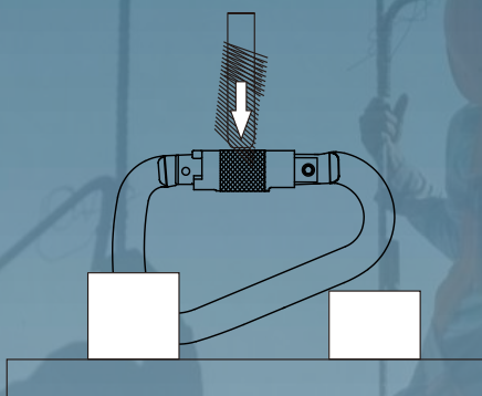
RESISTENCIA FRONTAL DEL GATILLO
