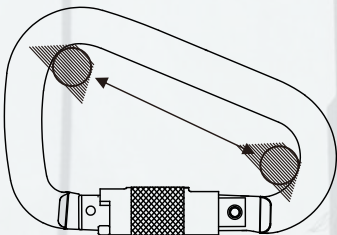
RESISTENCIA EN EJE MAYOR CON EL GATILLO CERRADO Y BLOQUEADO
